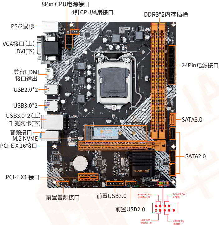
图1-1 B75 M.2主板图解
