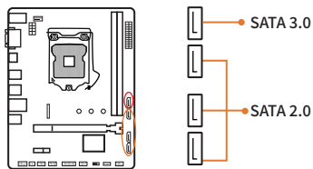
图2-10 SATA接口
